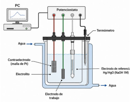
Figura 1. Esquema de la celda de 3 electrodos utilizada en los ensayos del paquete de trabajo 1.
