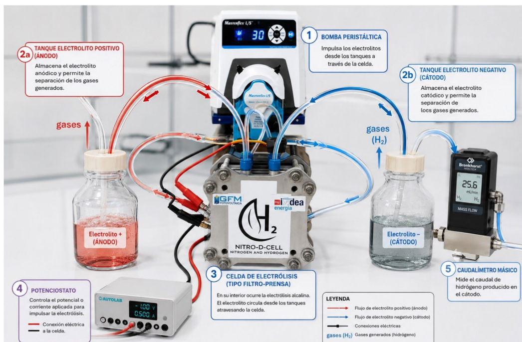
Figura 6. Prototipo de sistema de electrólisis Nitro D-Cell donde se desarrollaron los ensayos del paquete de trabajo 4.
